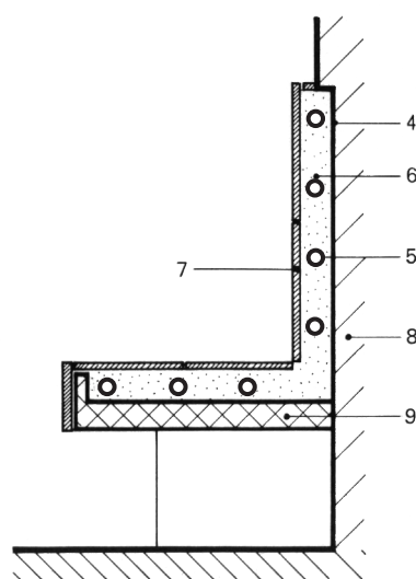
Schnitt durch Kachelaufbau mit Kachelplatten (2.)
