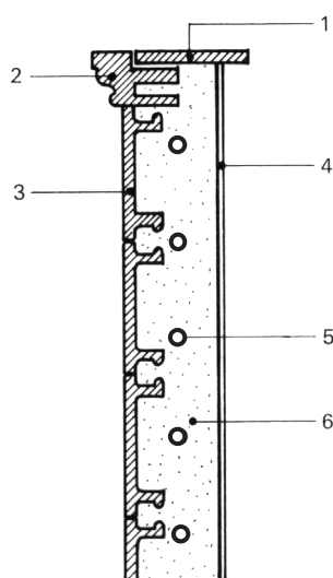
Schnitt durch Kachelaufbau mit Normalkacheln (1.)
